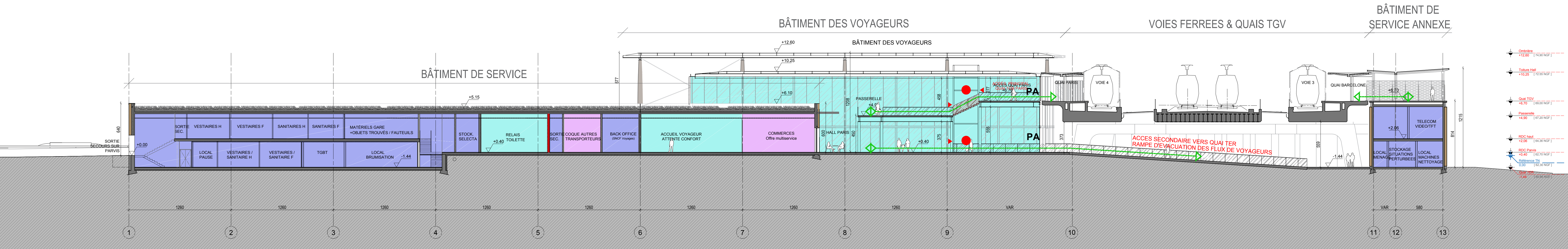
CPE 2 : Coupe longitudinale sur le bâtiment de service, les halls voyageurs et les voies TGV (Localisation sur la commune de Manduel)
