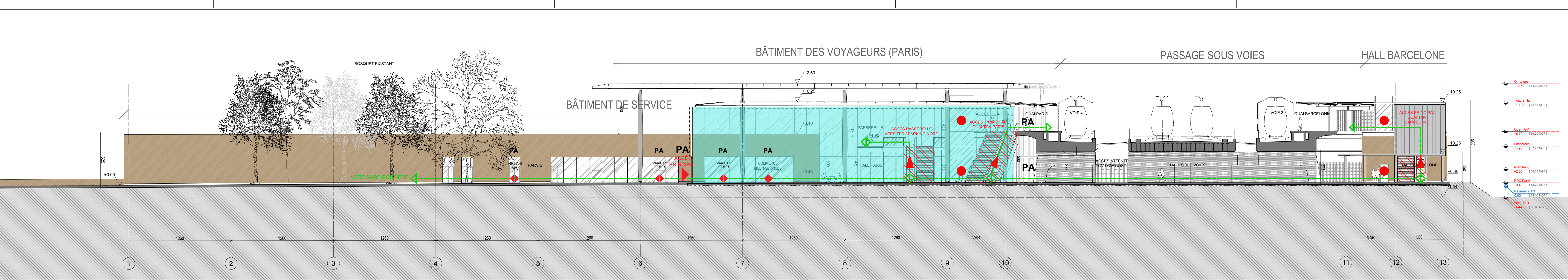
CPE 1 : Coupe longitudinale sur le parvis, les halls voyageurs et les voies TGV (Localisation sur la commune de Manduel)
