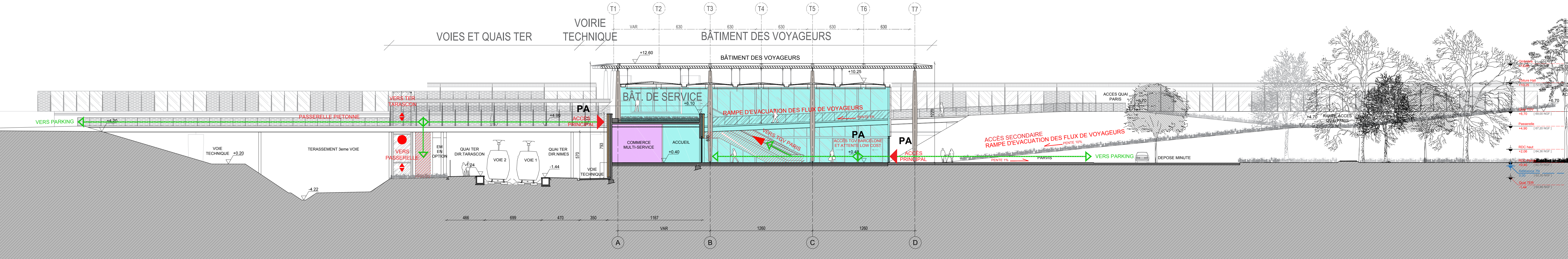
CPE 3 : Coupe transversale sur le bâtiment de service (1 niveau), le parvis et les voies TER (Localisation sur la commune de Manduel)
