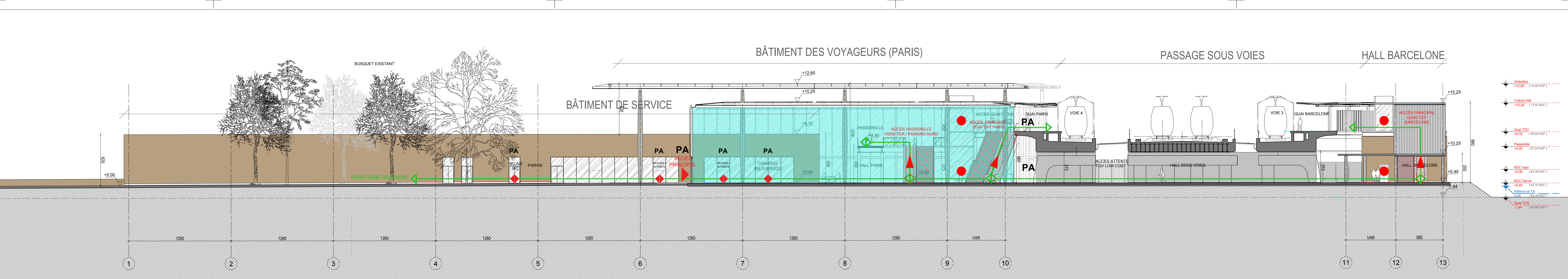
CPE 1 : Coupe longitudinale sur le parvis, les halls voyageurs et les voies TGV (Localisation sur la commune de Manduel)
